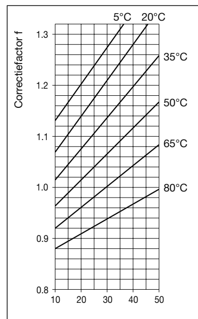
Gewichtsaandeel propyleenglycol [%]
