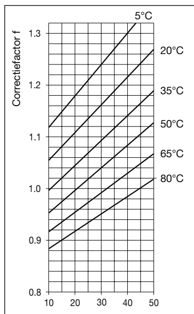
Gewichtsaandeel ethyleenglycol [%]
