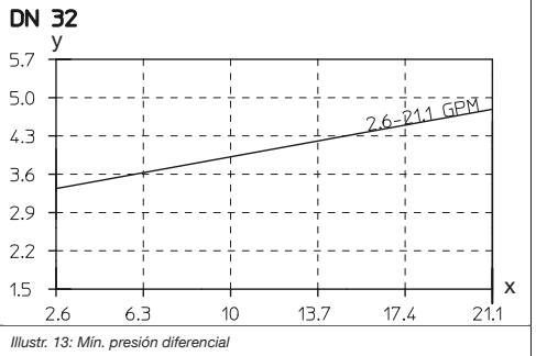
Ilustr. 13: Mín. presión diferencial
