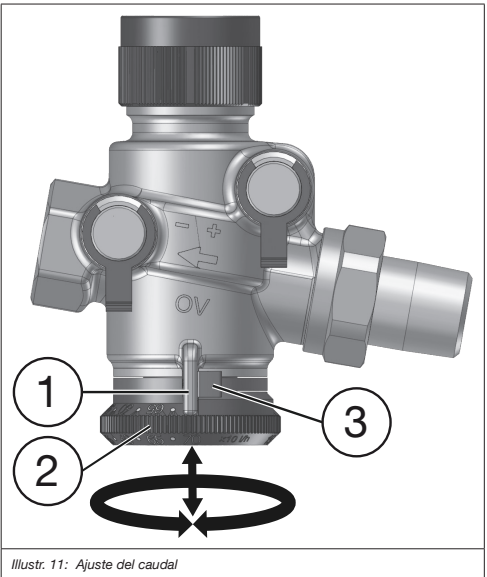
Ilustr. 11: Ajuste del caudal
