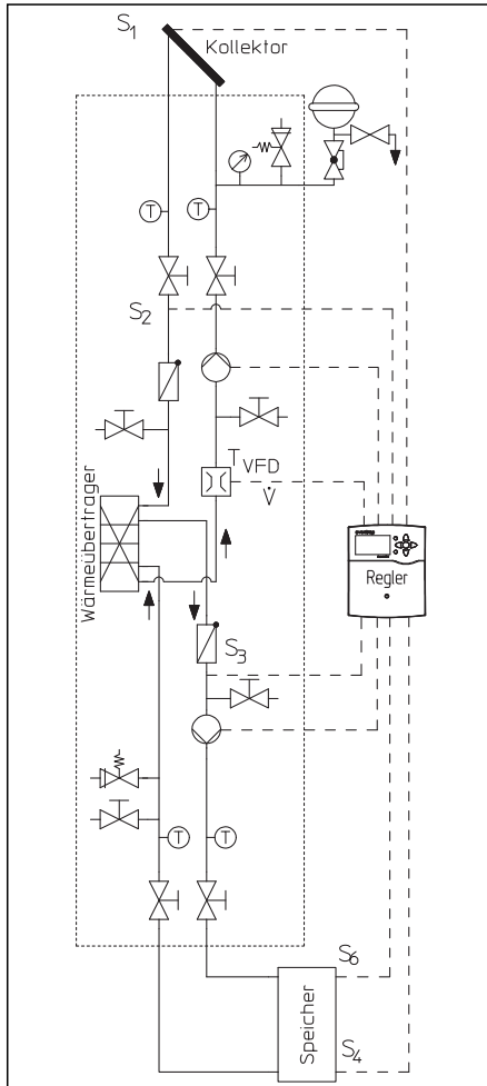
Abb. 23: Ausführung X-Uno
