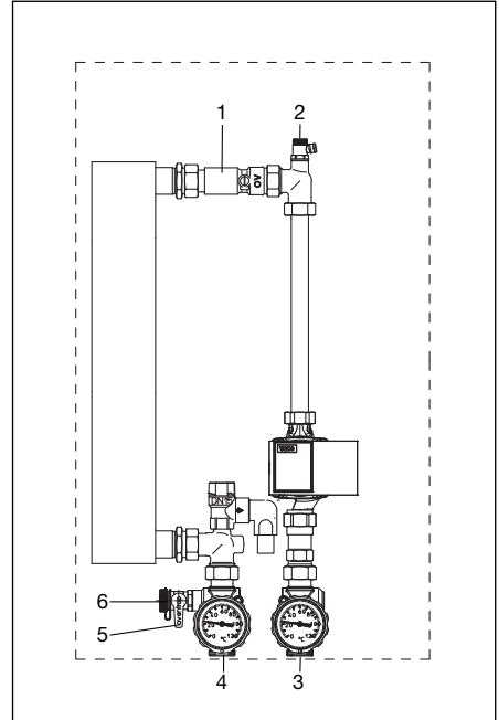
Illustr. 26: Remplissage, purge
