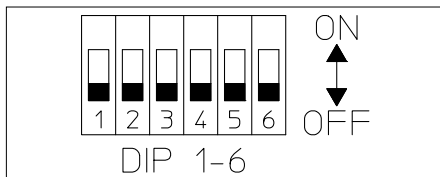
Abb. 6: Einstellung DIP-Schalter
