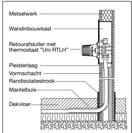
Doorsnede
