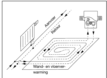
Inbouwtekening
