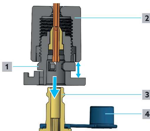
Ryc. 8: Podłączenie przewodu impulsowego do zaworu partnerskiego
