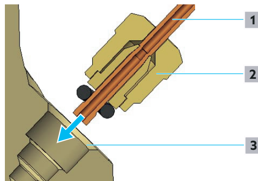
Afb. 7: Aansluiting pulsleiding op HydroControl D
