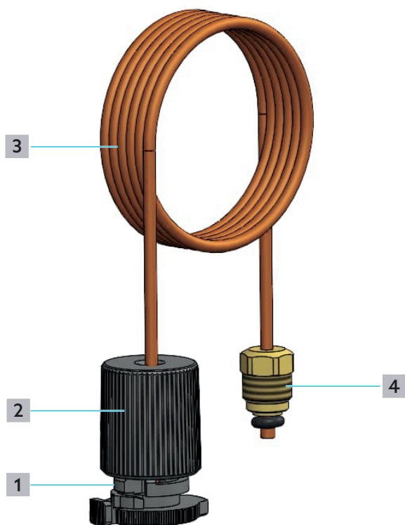
Obr. 6: Montáž impulzního vedení
