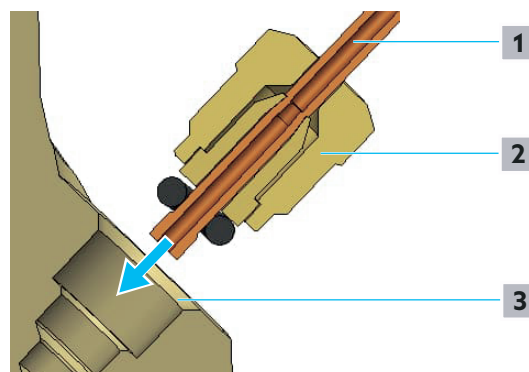
Fig. 7 - Collegamento della linea ad impulsi a HydroControl D
