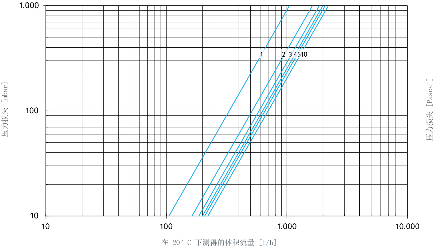
图 16: 体积流量预设置 DN 20
