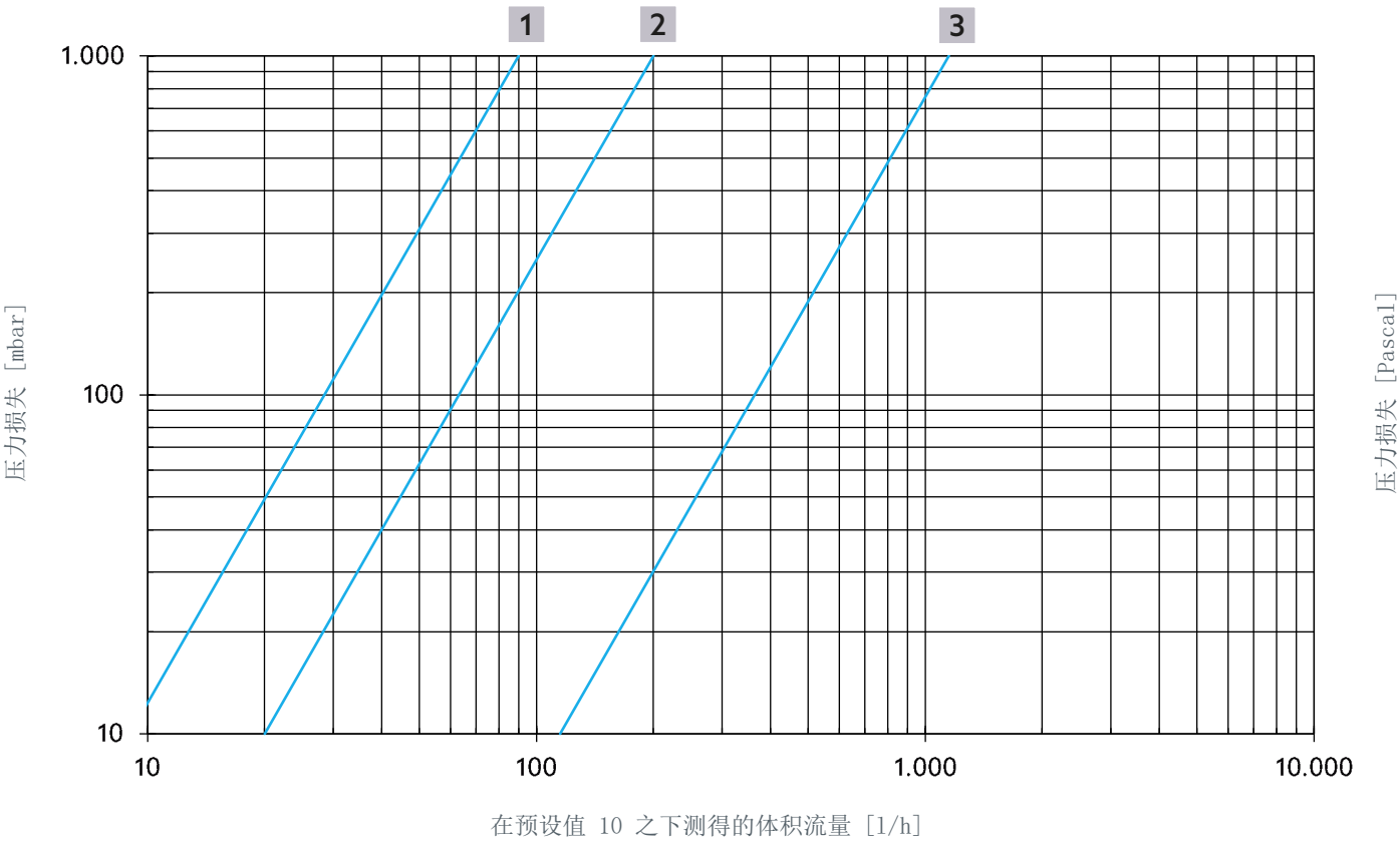
图 17: 产品编号 4202504 和 4202504, 4202604, 4202704, 4202804 的体积流量热力调节
