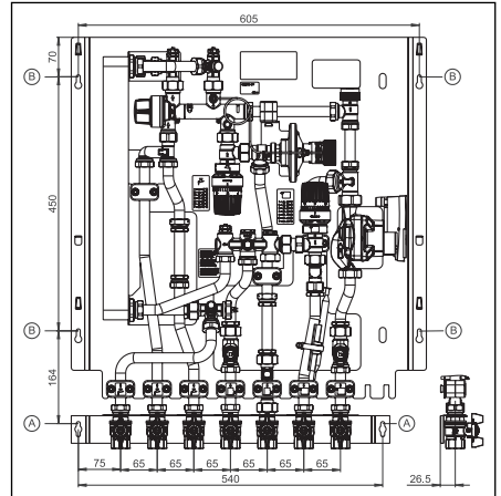
Abb. 5.5 Anschlussschema Kugelhahnanschlussleiste 1341180
