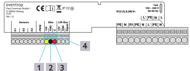
Abb. 9: Anschlussleiste Regumaq X-25
