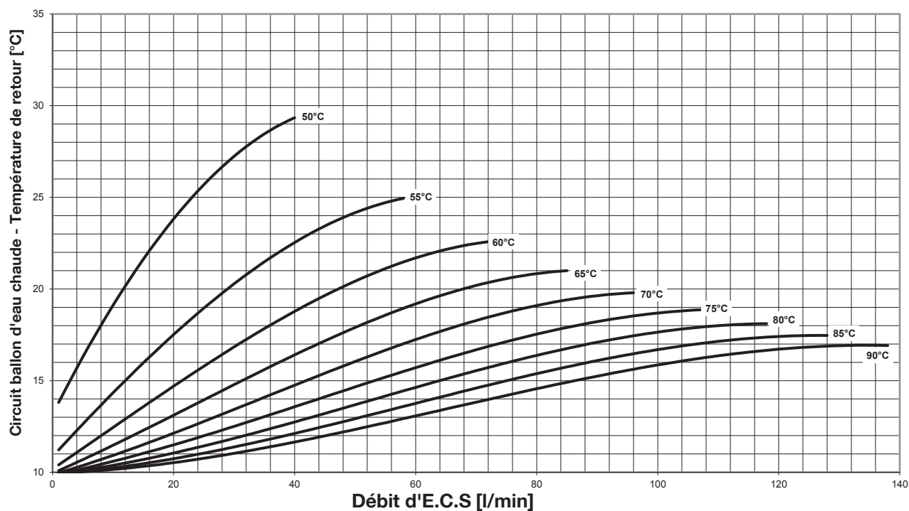
Température de retour circuit ballon d'eau chaude à différentes températures de départ - Réchauffage de l'eau potable de 10 °C à 50 °C -
