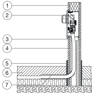
Abb. 8: Einbauquerschnitt
