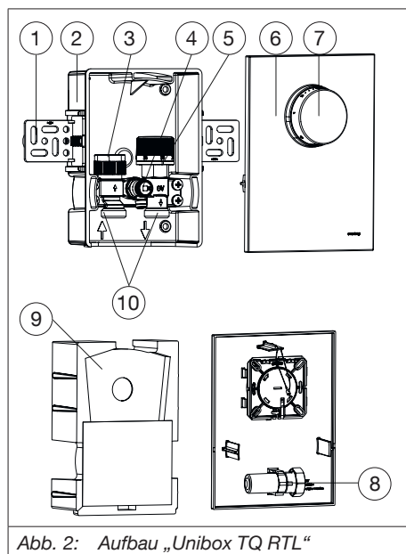
Abb. 2: Aufbau „Unibox TQ RTL“
