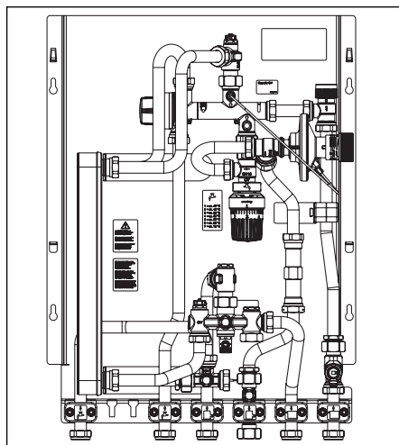
Afb. 1.1 “Regudis W-HTU”-woningstation
