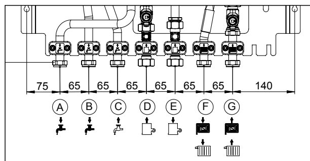
Dimensiuni racorduri
