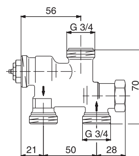
„TKM”-szelep (egycsöves/kétcsöves)
