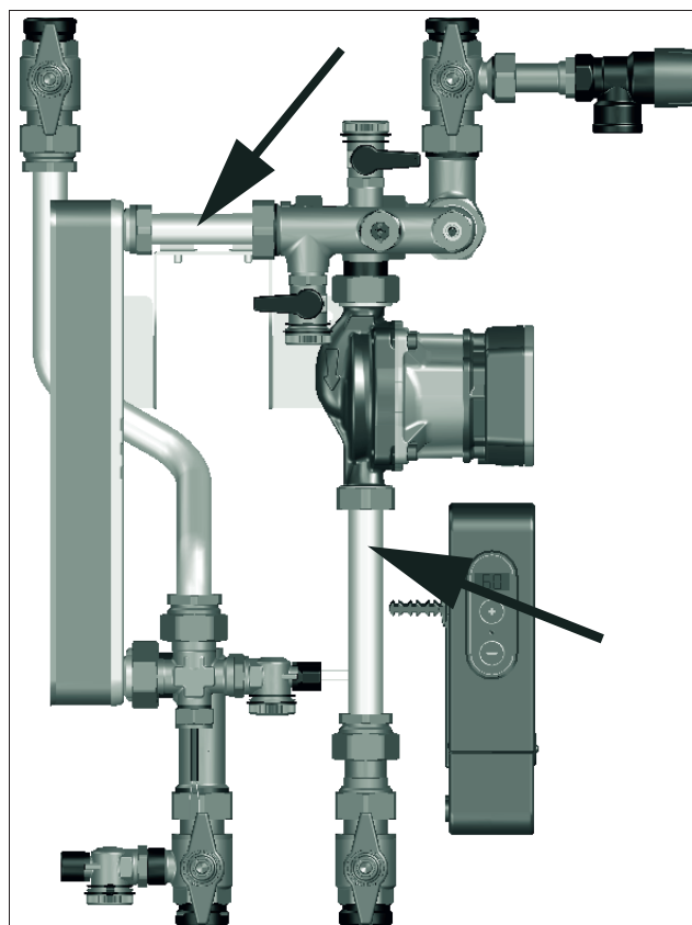
Fig. 19: Conexión equipotencial
