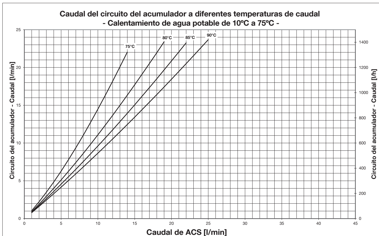
Fig. 57: Caudal del circuito primario- calentamiento de agua potable hasta 75 °C
