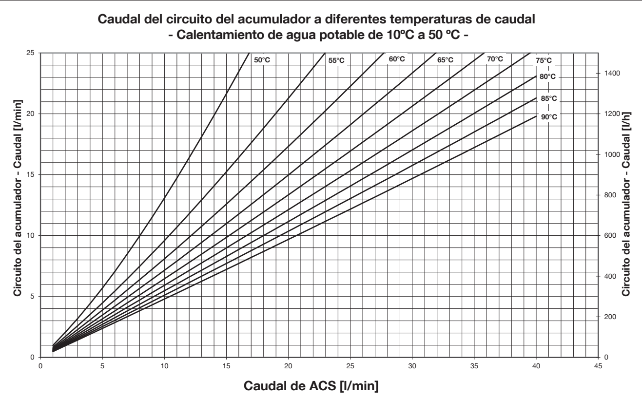
Fig. 47: Caudal del circuito primario– calentamiento de agua potable hasta 50 °C
