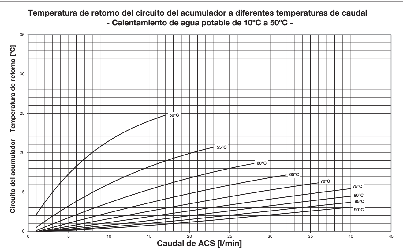
Fig. 48: Temperatura de retorno del circuito primario– calentamiento de agua potable hasta 50 °C
