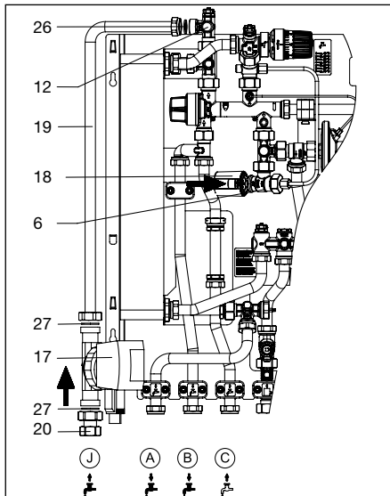
Abb. 6.1 Montage
