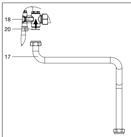
Fig. 6.4 Assemblaggio / Rimozione
