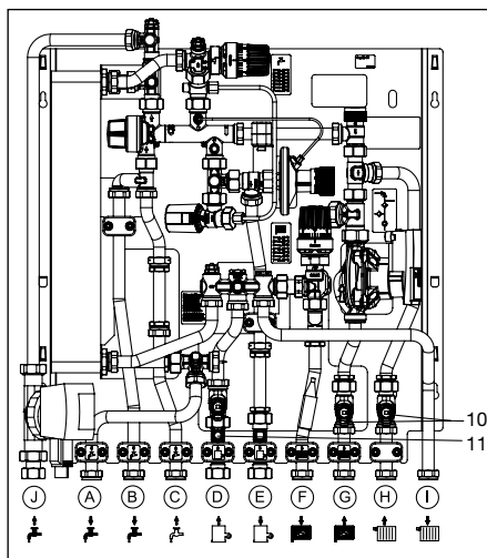
Abb. 8.1 Einbauposition Schmutzfänger
