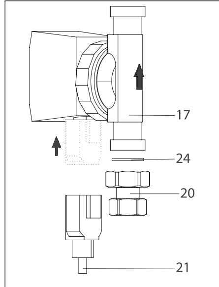
Abb. 6.2 Pumpenausrichtung
