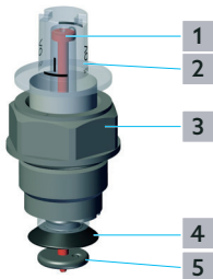
Abb. 1: Aufbau Durchflussindikator
