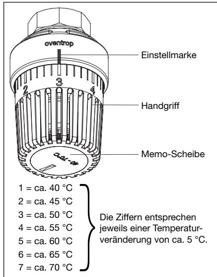
Abb. 8.4 Einstellung Trinkwassertemperatur
