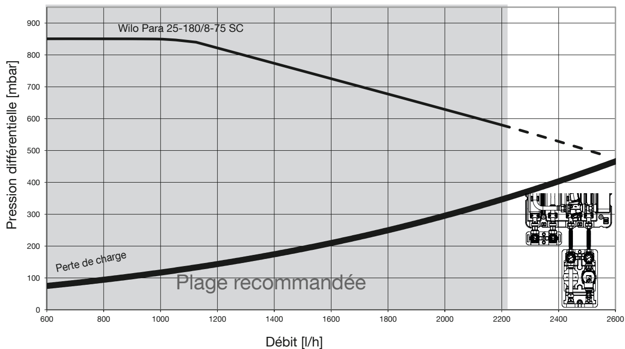
Fig. 5: Perte de charge circuit secondaire Regudis H-H
