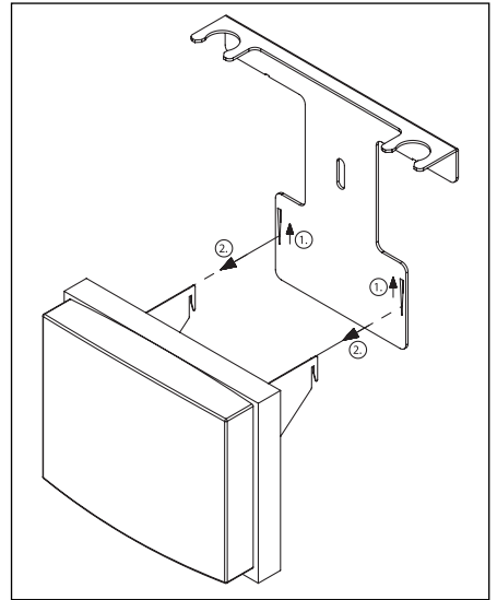
Abb. 16 Demontage Blinddeckel mit Halteblech
