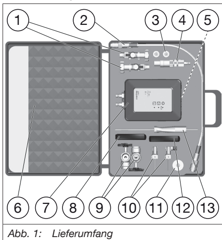
Abb. 1: Lieferumfang
