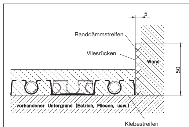
Maße Randdämmstreifen
