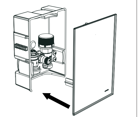
Abb. 10: Abdeckung aufsetzen
