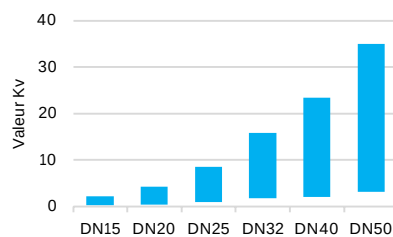
Plages de débit DN 15 à DN 50
