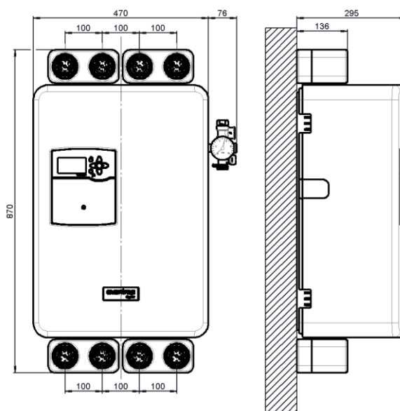
Abb. 9: „Regudis H-HT“ mit Kugelhahnanschluss Sets
