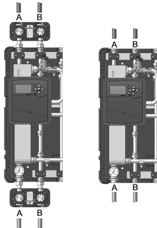
Abb. 17: Primärseitiger Anschluss der Versorgungsleitungen (Vorlauf = A; Rücklauf = B) entweder von oben oder von unten.
