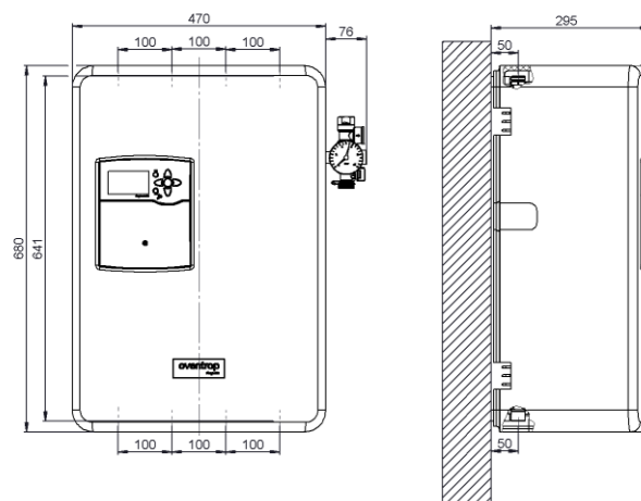
Abb. 8: Abmessungen „Regudis H-HT“
