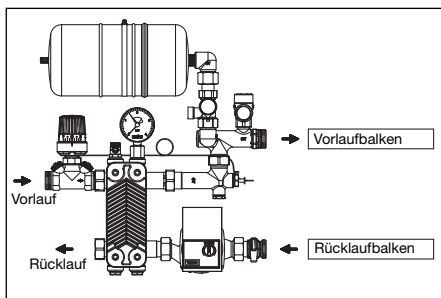
Abb. 6.2 Durchflussrichtung
