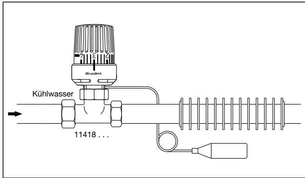
System-Darstellung Zweileiter-System Kälte
