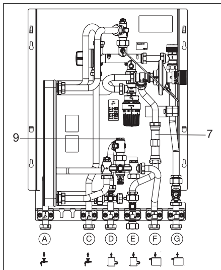
Afb. 6.1 Inbouw warmtemeter
