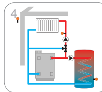
Mieszany obieg grzewczy z nagrzewaniem wody użytkowej
