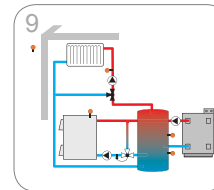
Mieszany obieg grzewczy z kotłem na paliwo stałe i ogrzewaniem dodatkowym
