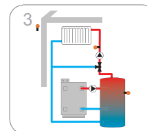
Mieszany obieg grzewczy z ogrzewaniem dodatkowym i pompą ładowania
