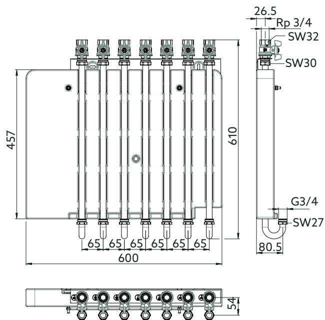
Fig. 2: Dimensions
