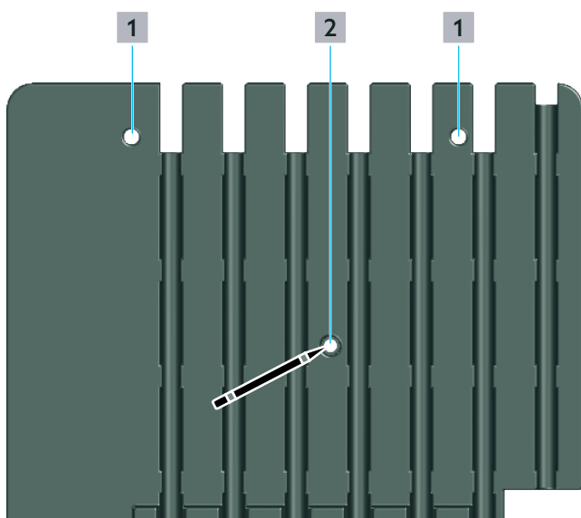
Fig. 7: Fixarea izolației
