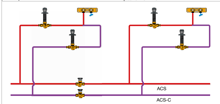
Figura del sistemas de las válvulas para empotrar "Aquastron"
