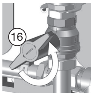
Fig. 5.9: Ouvrir le robinet d'arrêt à tournant sphérique sur l'aller du circuit primaire
