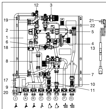
Fig. 5.1 Struttura con circuito di riscaldamento diretto e riciccolo
