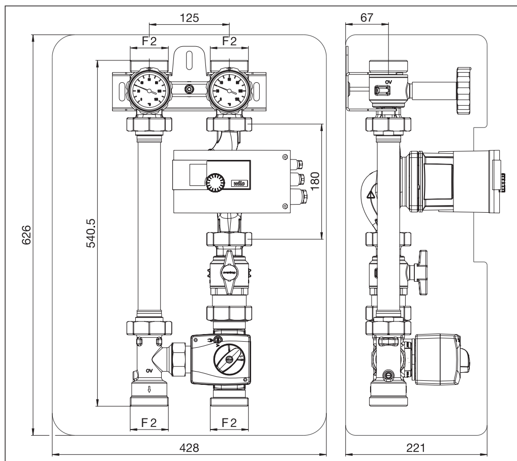
Dimensiuni „Regumat M3-180 plus“ DN 32
