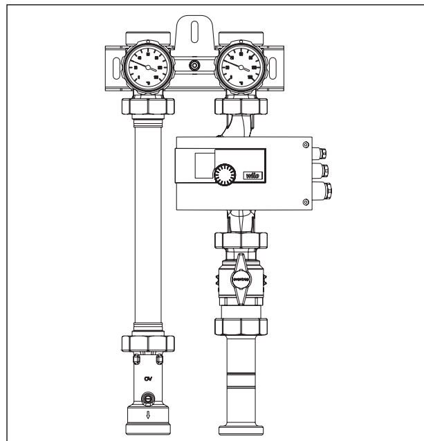
„Regumat S-180 plus“ DN 32 cu robinet sferic pentru pompă
