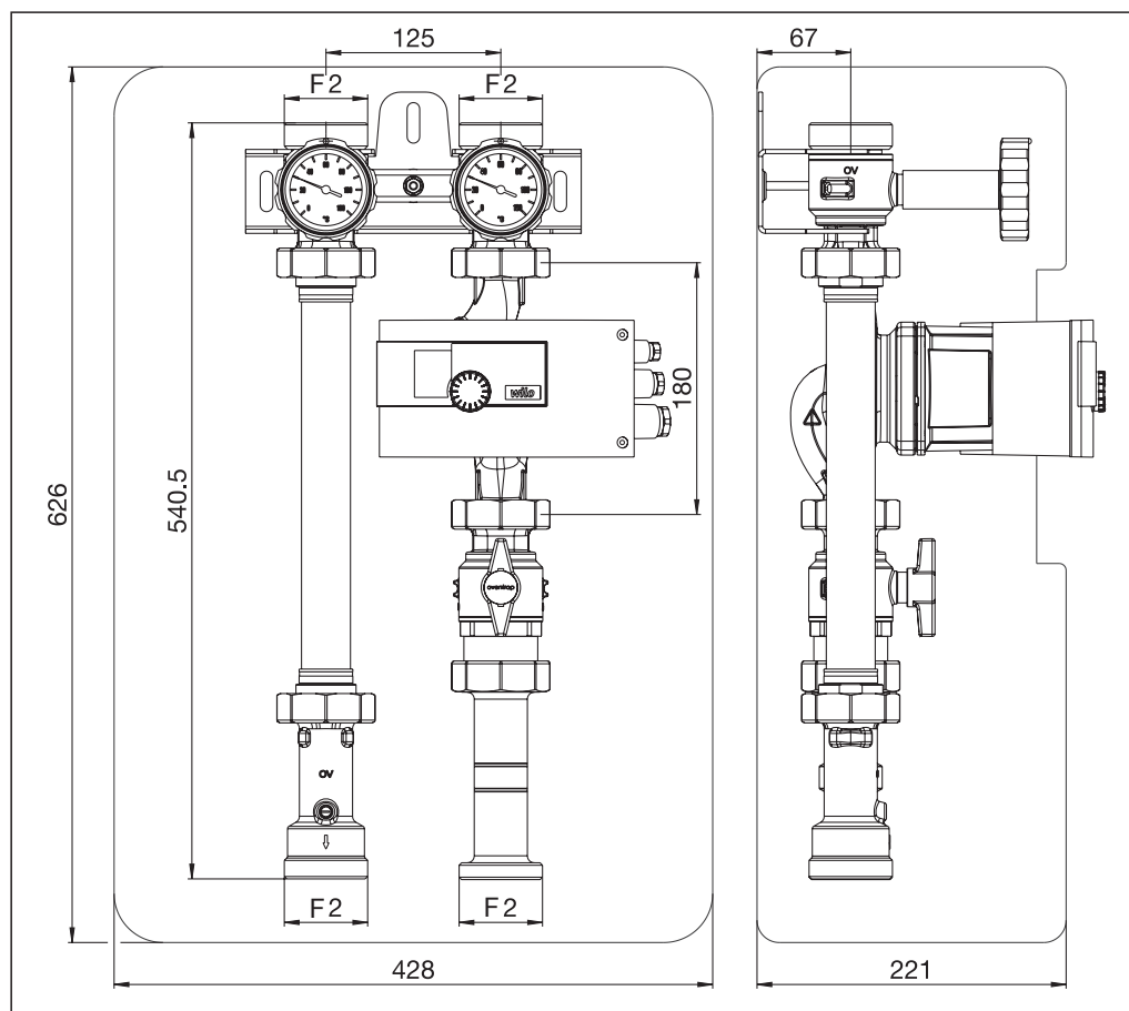
Dimensiuni „Regumat S-180 plus“ DN 32
