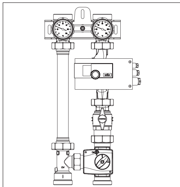
„Regumat M3-180 plus“ DN 32 cu robinet sferic pentru pompă
