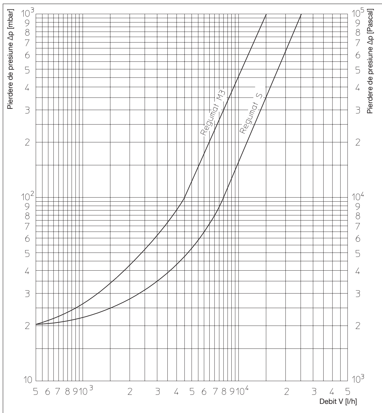
Diagramă de debit
