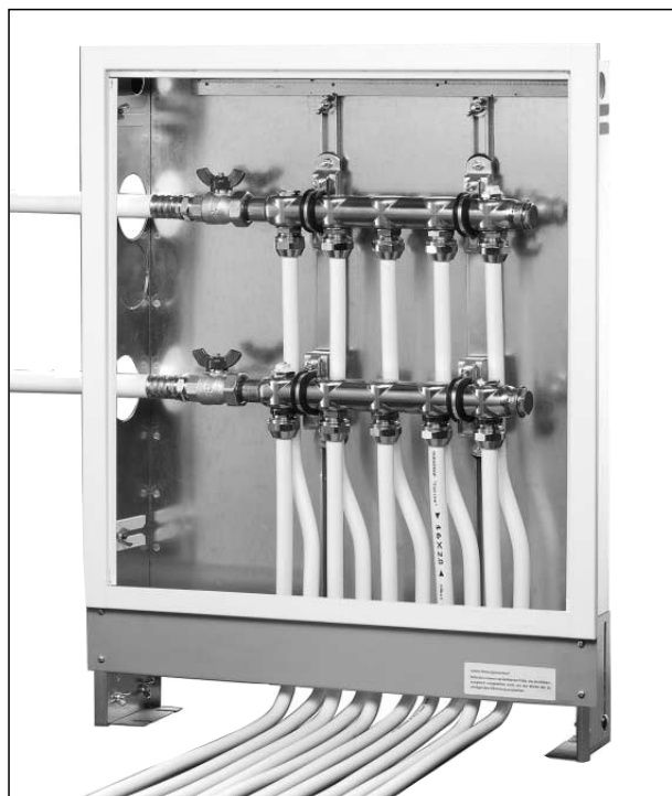
Distributeur/collecteur «Multidis SH» en acier inoxydable
