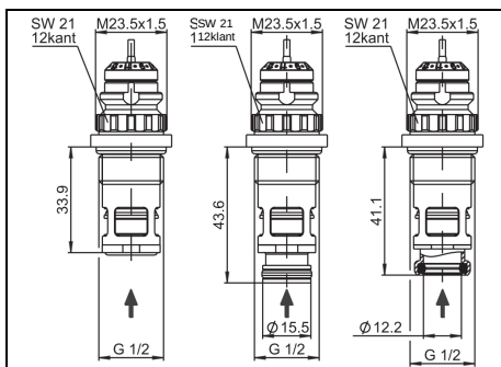
Afb. 2: Afmetingen en doorstroomrichting type GDQ
