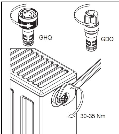
Afb. 3: Montage schuifafsluiter
