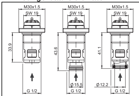
Afb. 1: Afmetingen en doorstroomrichting type GHQ
