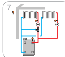
Un circuit de încălzire mixt și unul nemixt cu postîncălzire
