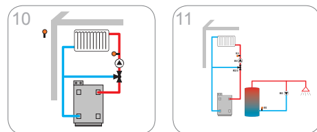
Un circuit de încălzire mixt cu senzor exterior central (Slave)
