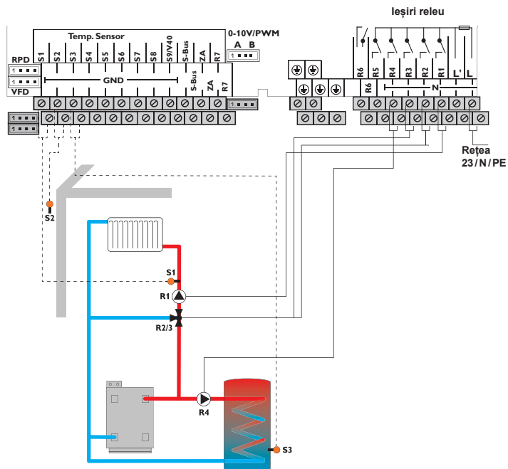
Schema 4: un circuit de încălzire mixt cu încălzirea apei menajere
