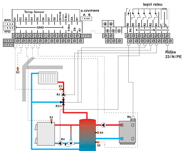
Schema 9: un circuit de încălzire mixt cu cazan de combustibil solid și postîncălzire (Cerere)
