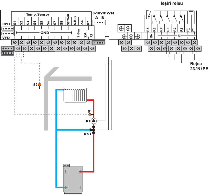
Schema 1: un circuit de încălzire mixt
