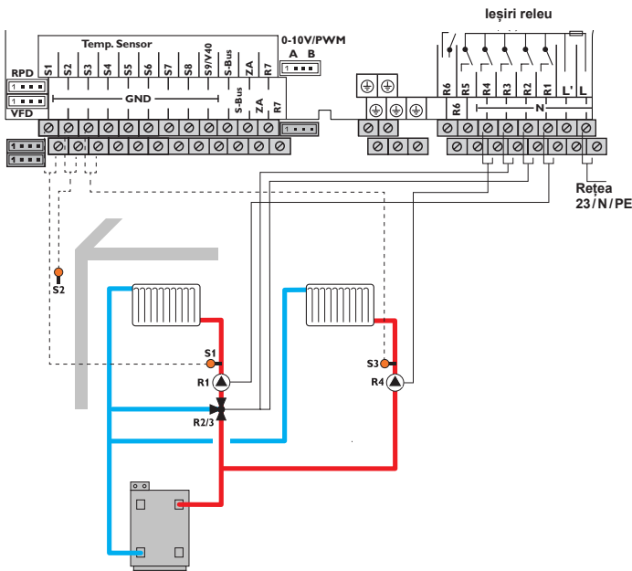
Schema 6: un circuit de încălzire mixt și unul nemixt
