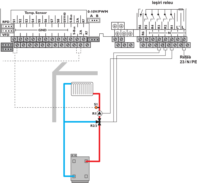
Schema 10: un circuit de încălzire mixt cu senzor central pentru temperatura exterioră (Slave 2...20)
