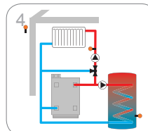
Un circuit de încălzire mixt cu încălzirea apei de consum
