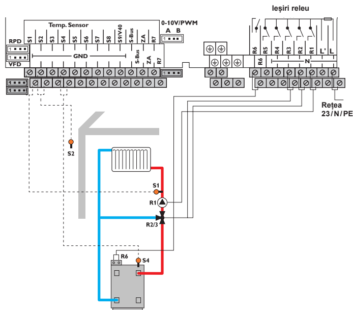
Schema 2: un circuit de încălzire mixt cu postîncălzire (Cerere)
