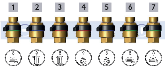
Abb. 2: Anschlussbelegung
