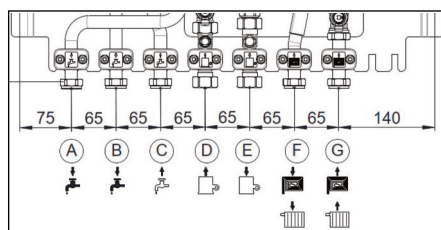
Fig. 4.3 Dimensioni collegamenti
