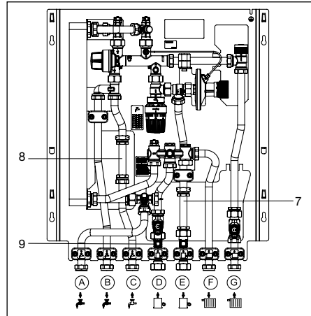
Abb. 6.1 Einbau Kaltwasser- und Wärmezähler
