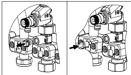
Fig. 6.5 Montaggio tappi
