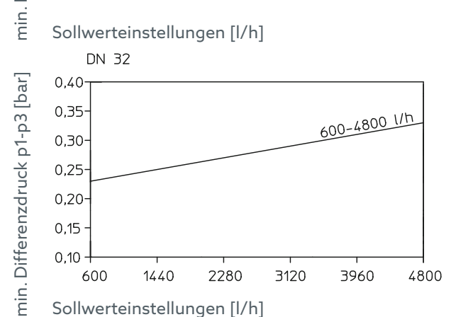
Abb. 13: Mindest-Differenzdrücke
