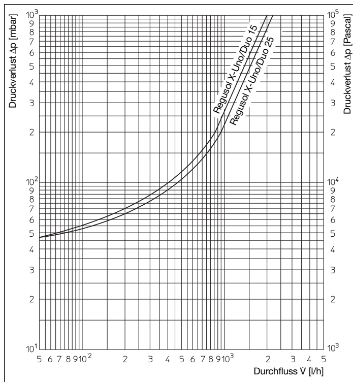
Abb. 6.1 Durchflussdiagramm
