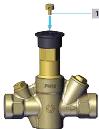
Ryc. 7: Zablokowanie wartości zadanej temperatury
