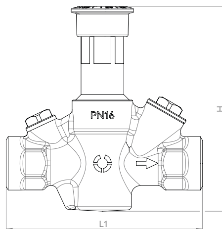
Fig. 2: Encombres latéraux
