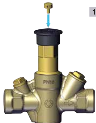
Fig. 7: Bloquear el valor prefijado de temperatura
