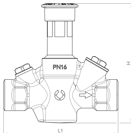
Рис. 2: Размеры сбоку
