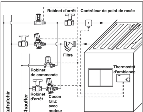
Fig. 7: Exemple de montage 1: Système a quatre tuyaux
