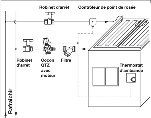
Fig. 6: Exemple de montage 1: Système a deux tuyaux
