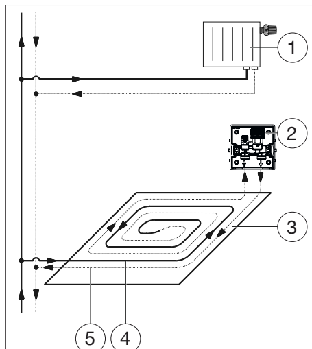
Abb. 6: Anschluss
