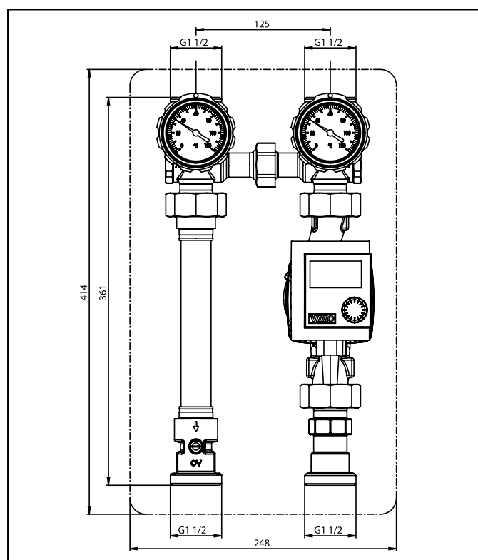
Рис. 4.4 „Regumat S-180“ DN 25
