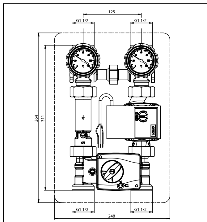
Рис. 4.3 „Regumat M4-130“ DN 25
