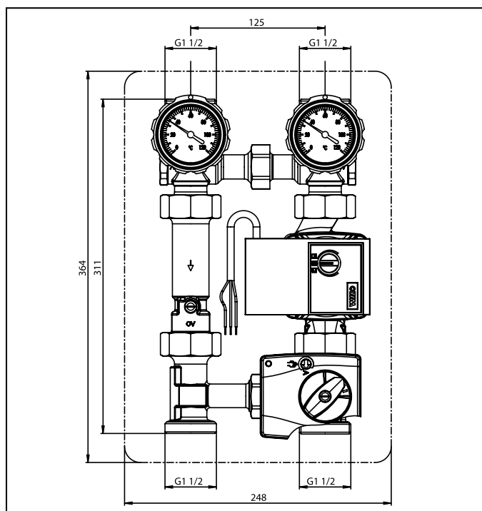
Рис. 4.2 „Regumat M3-130“ DN 25
