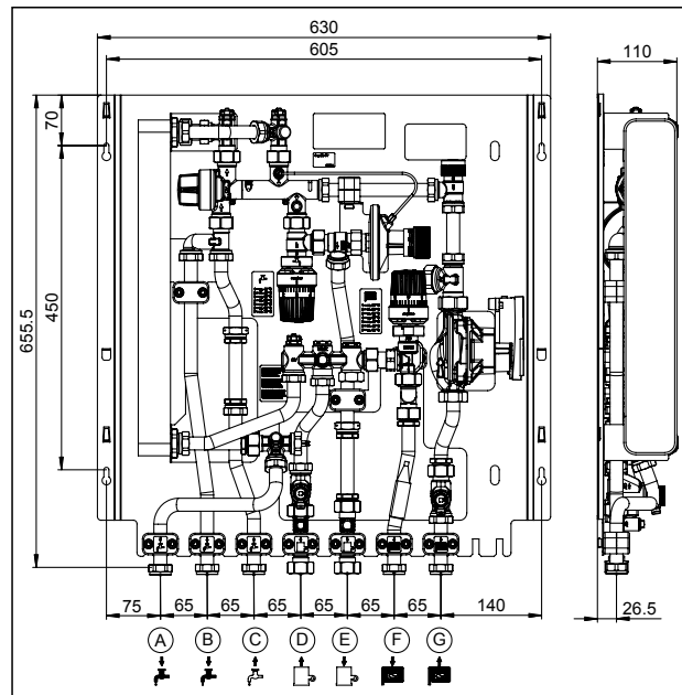
Abmessungen mit gemischtem Heizkreis
