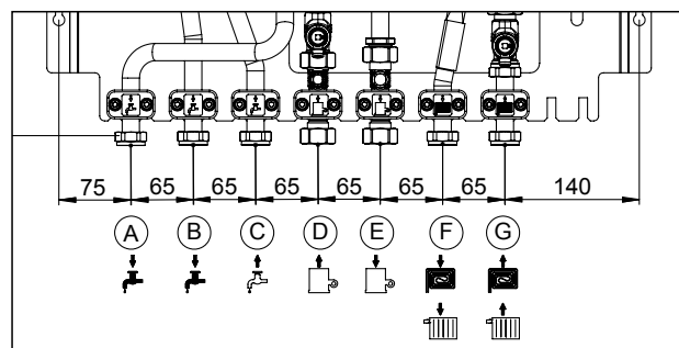
Anschlussmaße
