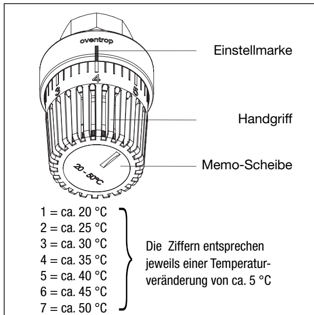
Temperaturregler
