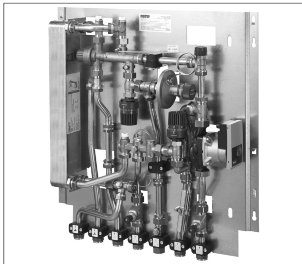
„Regudis W-HTF“ - gemischter Heizkreis
