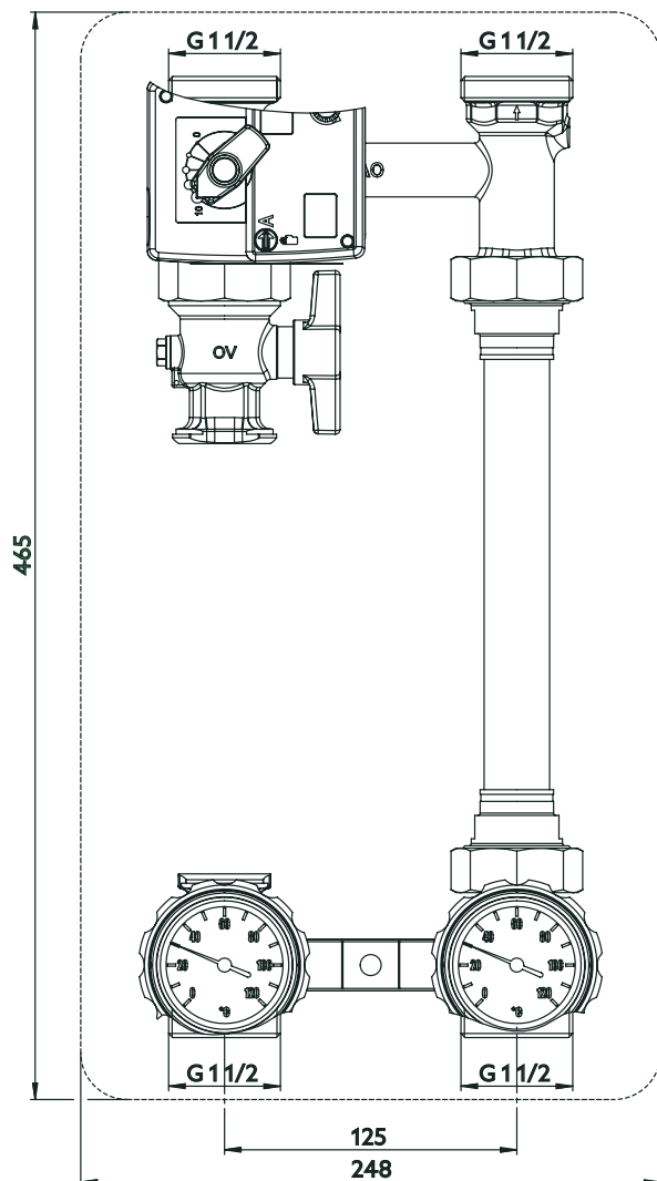
Abb. 20: Vorderansicht
