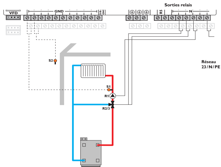
Schéma 1: circuit de chauffage mélangé
