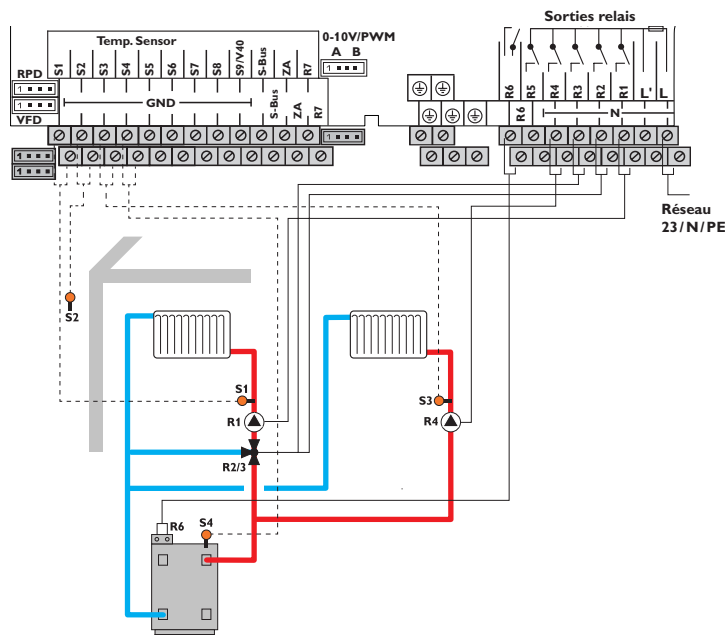
Schéma 7: circuit de chauffage mélangé et circuit de chauffage direct avec chauffage d'appoint (demande)
