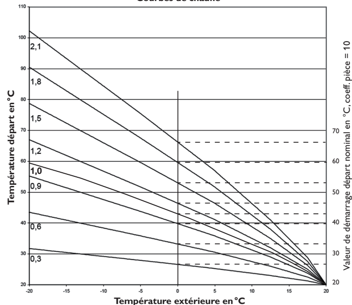
Courbes de chauffe
