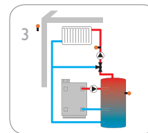
Circuit de chauffage mélangé avec chauffage d'appoint et pompe de charge
