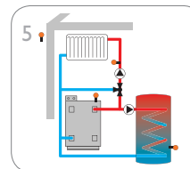
Circuit de chauffage mélangé avec chauffage de l'ECS et chauffage d'appoint
