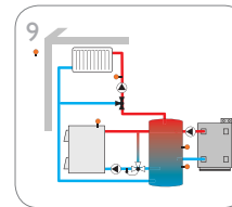
Circuit de chauffage mélangé avec chaudière à combustible solide et chauffage d'appoint
