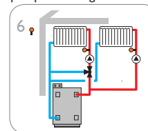
Circuit de chauffage mélangé et circuit de chauffage direct
