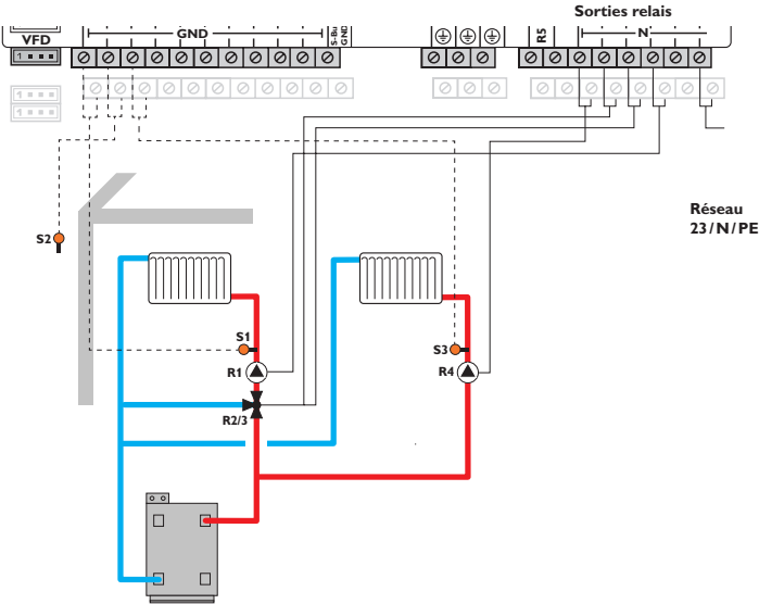
Schéma 6: circuit de chauffage mélangé et circuit de chauffage direct
