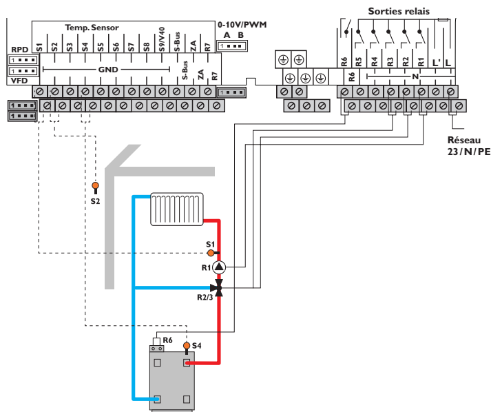
Schéma 2: circuit de chauffage mélangé avec chauffage d'appoint (demande)
