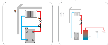
Circuit de chauffage mélangé avec sonde extérieure centrale (esclave)
