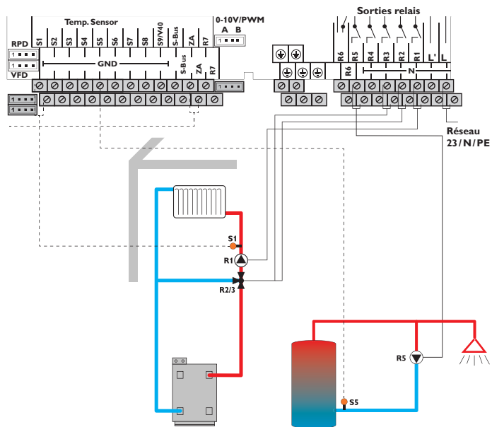
Schema 11: circuit de chauffage mélangé avec sonde extérieure centrale et circulation (esclave 2...20)
