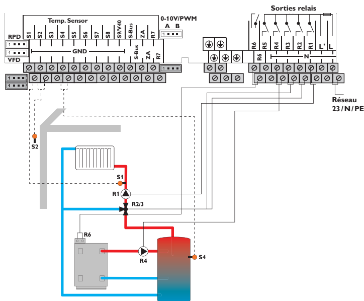
Schéma 3: circuit de chauffage mélangé avec chauffage d'appoint (demande ou pompe de charge de la chaudière)
