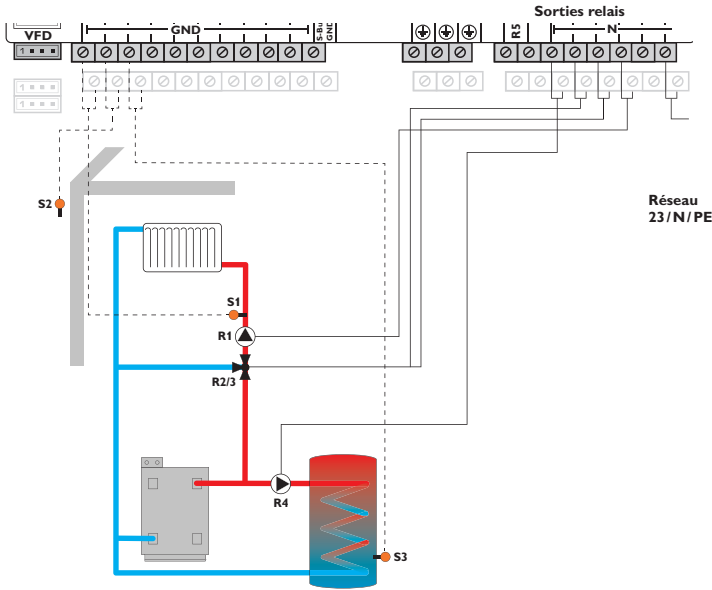
Schéma 4: circuit de chauffage mélangé avec chauffage de l'ECS
