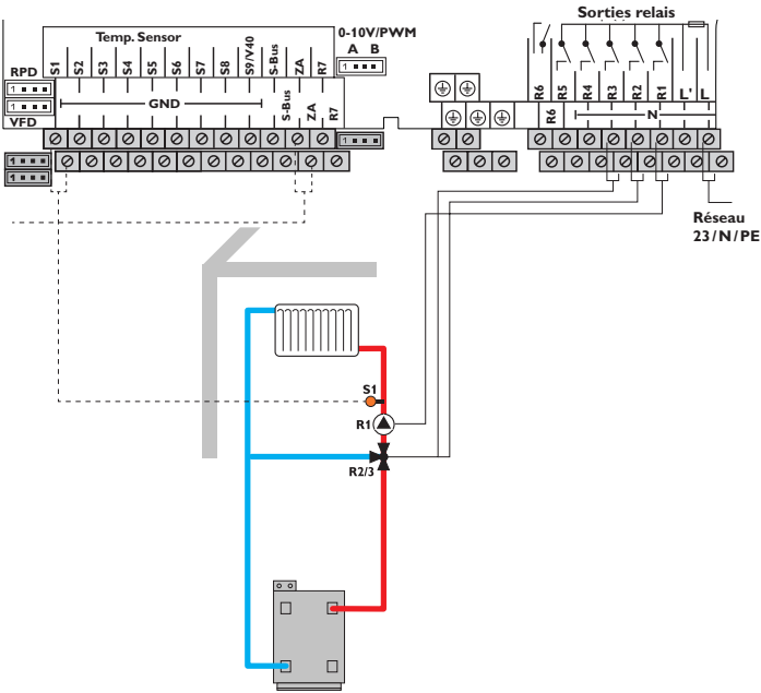
Schéma 10: circuit de chauffage mélangé avec sonde extérieure centrale (esclave 2... 20)
