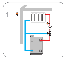
Circuit de chauffage mélangé
