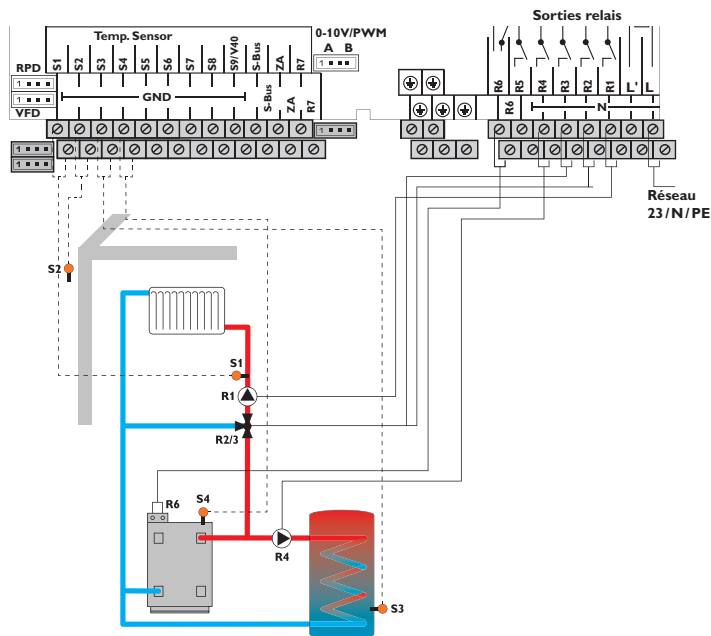
Schéma 5: circuit de chauffage mélangé avec chauffage de l'ECS et chauffage d'appoint (demande pour le circuit de chauffage et l'ECS)
