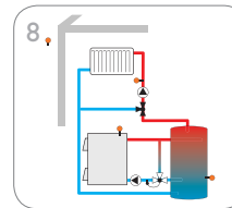
Circuit de chauffage mélangé avec chaudière à combustible solide
