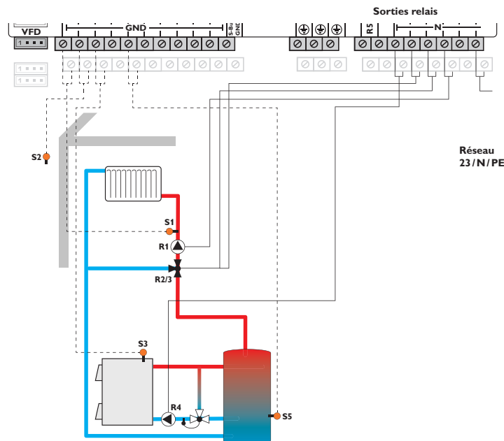
Schéma 8: circuit de chauffage mélangé avec chaudière à combustible solide
