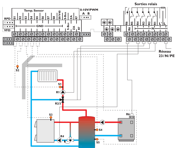
Schéma 9: circuit de chauffage mélangé avec chaudière à combustible solide et chauffage d'appoint (demande)
