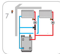
Circuit de chauffage mélangé et circuit de chauffage direct avec chauffage d'appoint
