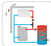
Circuit de chauffage mélangé avec chauffage de l'ECS
