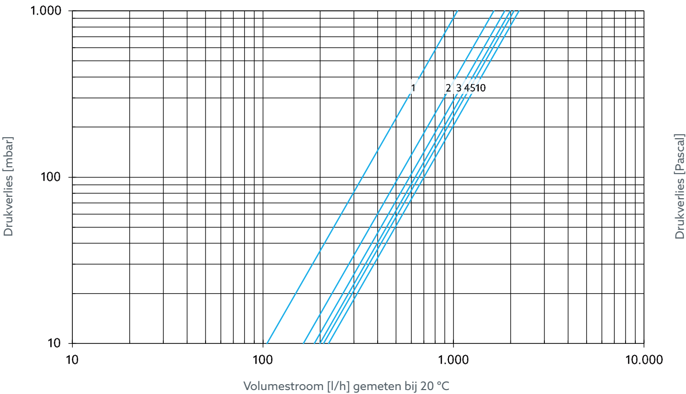
Afb. 16: Voorinstelling volumestroom DN 20
