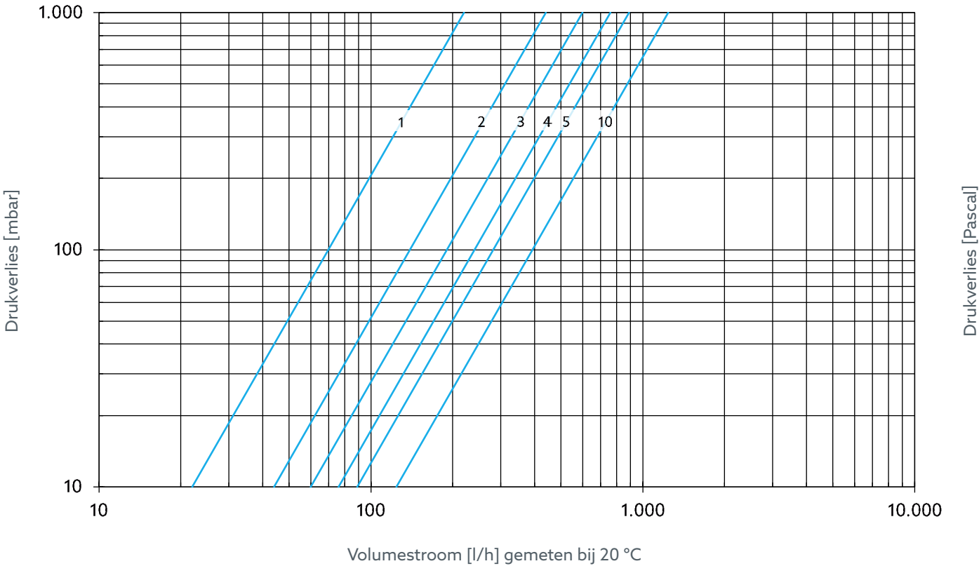
Afb. 15: Voorinstelling volumestroom DN 15
